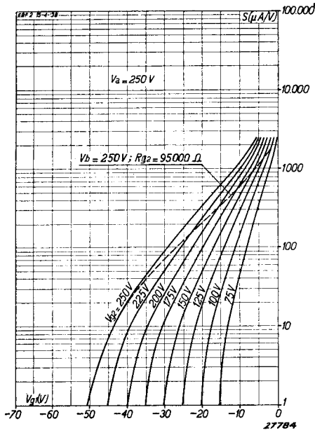
Abb. 4 S/V_{g_1} -Kurvenschar der EBF 2 mit V_{g_1} als Parameter. Die gestrichelte Kurve gibt den Verlauf der Steilheit bei Regelung der Röhre für den Fall der Speisung des Schirmgitters über einen Vorwiderstand von 95.000 \Omega von 250 Volt aus.
