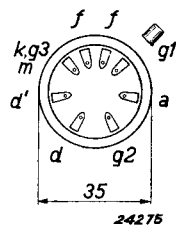
Abb. 2 Elektrodenanordnung und Sockelanschlüsse.
